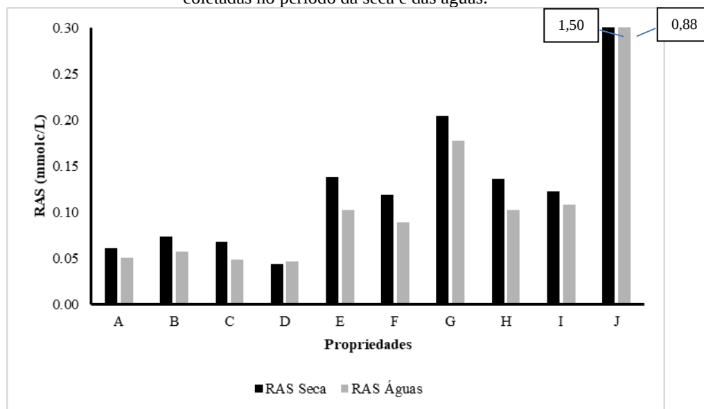
Figura 3. Valores da Relação de Adsorção de Sódio para efeito comparativo entre o resultado das amostras coletadas no período da seca e das águas.
