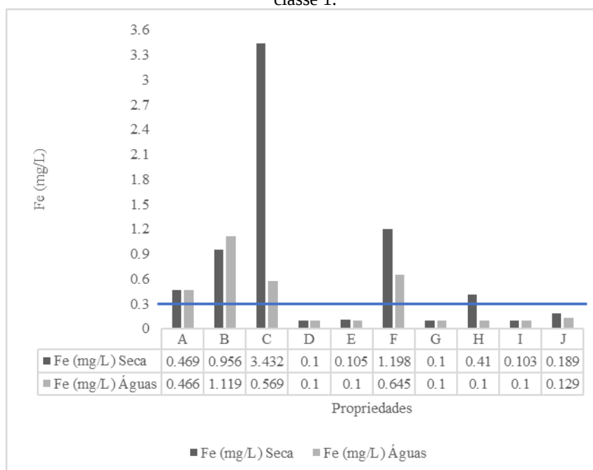
Figura 5. Valor de referência para Fe estabelecido pela resolução nº 357 do CONAMA para águas doces de classe 1.
