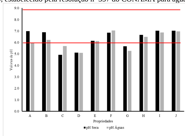
Figura 1. Potencial hidrogeniônico (pH) da água no período seco e chuvoso das propriedades e faixa ideal de pH entre 6,0 e 9,0, estabelecido pela resolução nº 357 do CONAMA para águas doces de classe 1.
