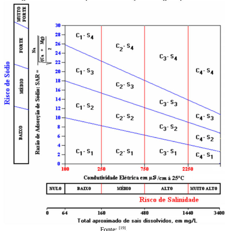
Figura 4. Diagrama de Richards para classificação das águas para fins de irrigação.
